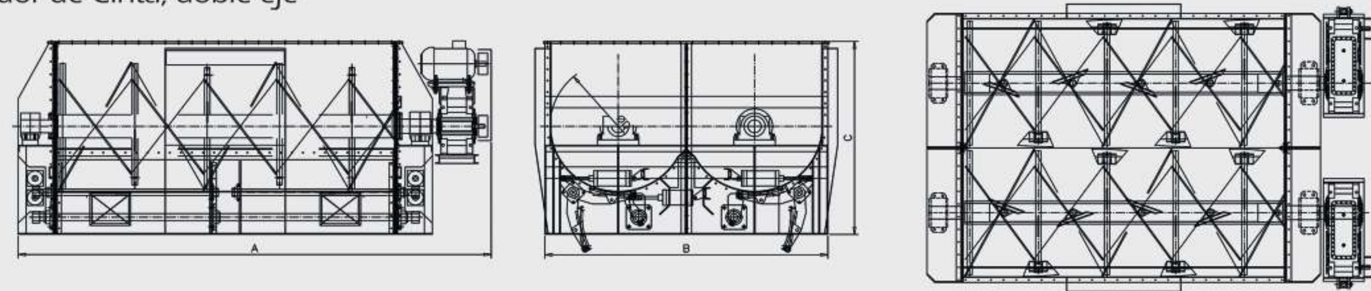
Mezclador de Cinta, doble eje
