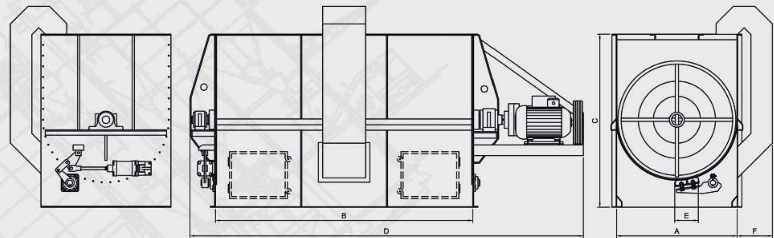
Mezclador de Cinta, un solo eje
